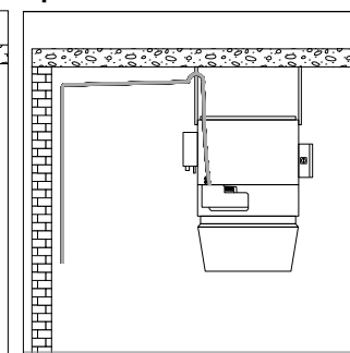
TopVent® TP
