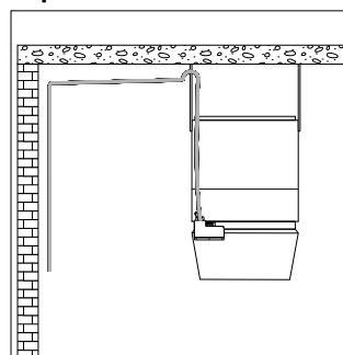
Kép: Kondenzátum-elvezetés
