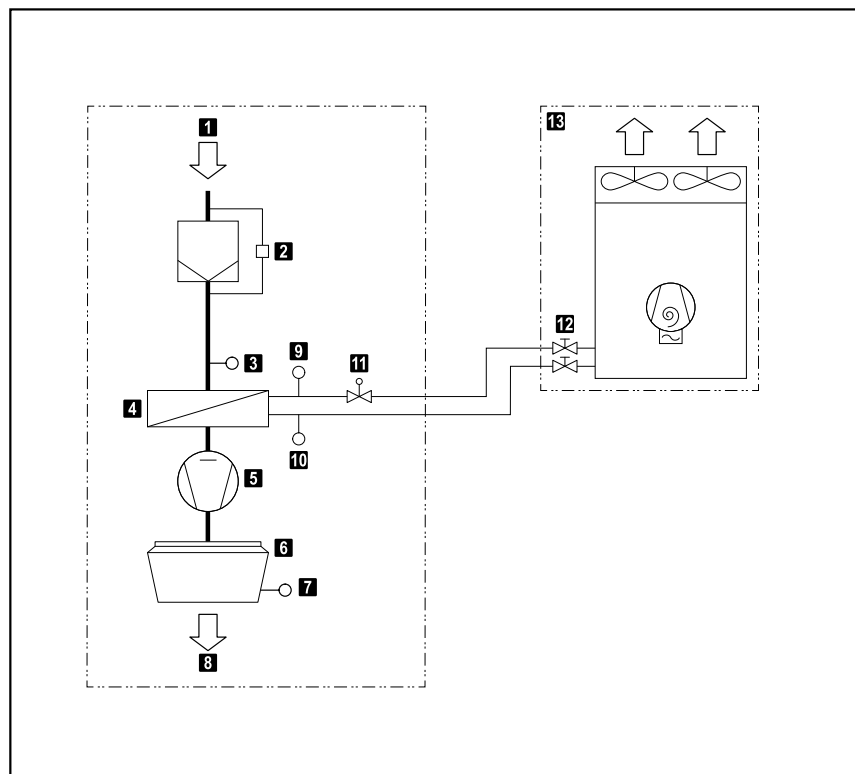
Táblázat: TopVent® TPH-11P működési vázlata
