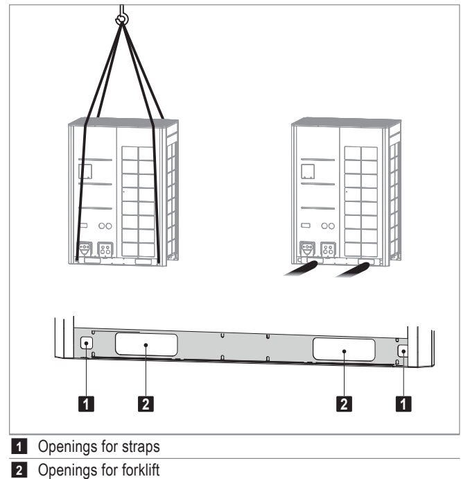
Fig. E1: Lifting the heat pump
