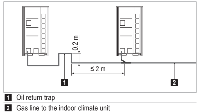
Fig. E11: Oil return trap
