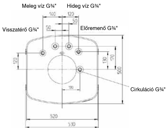
Felülnézet „X”
