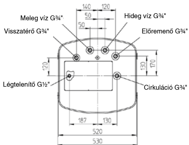
Felülnézet „X”
