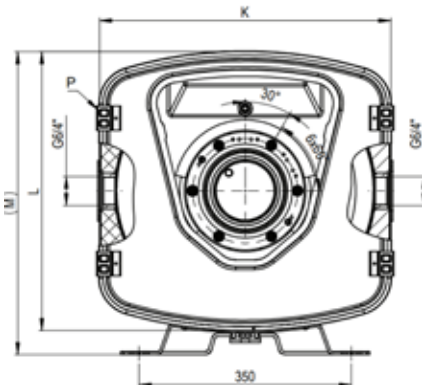
Felülnézet
