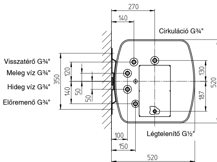
Alulnézet „X”
