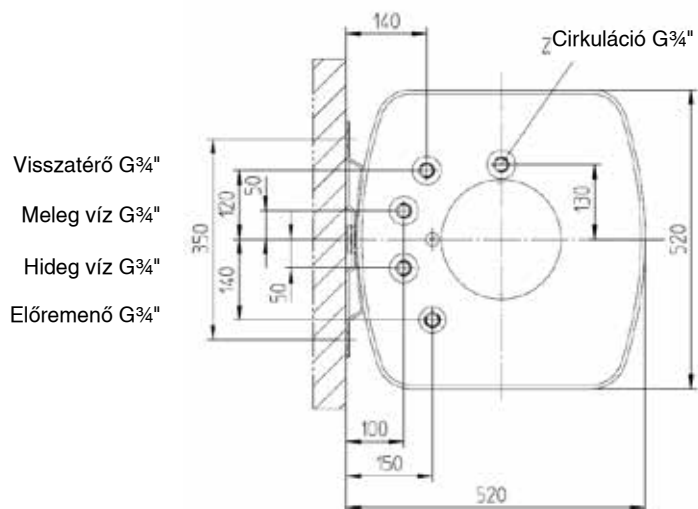
Alulnézet „X”
