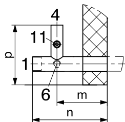
Metszet A
