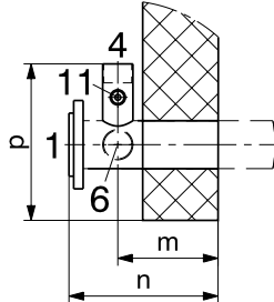
Metszet B
