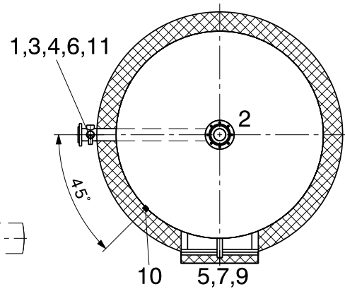
Metszet B
