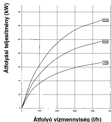
Átfolyási teljesítmény (60 °C) S 1500 PR - 3,6 m 2
