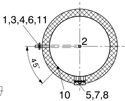
Metszet A
