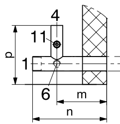
Metszet A
